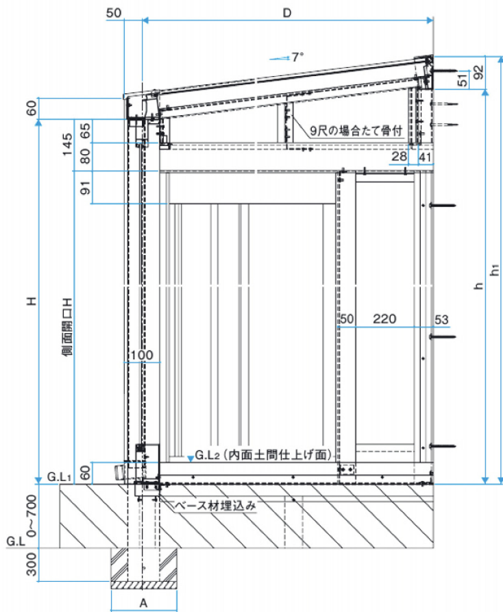
●C-C' 断面
