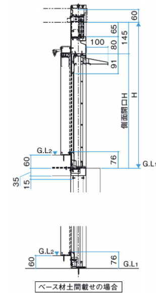
●A-A' 断面
