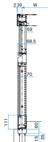
●B-B' 断面
