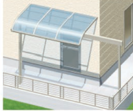
梁置き納まり |R型|F型|
